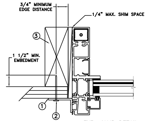
TYP. JAMB DETAIL HORIZONTAL SECTION
